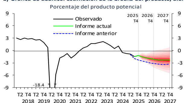
b) Gráfica de abanico: estimación de la brecha del producto, a.e. 1/
